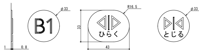
押ボタン意匠 (1 : 2)
