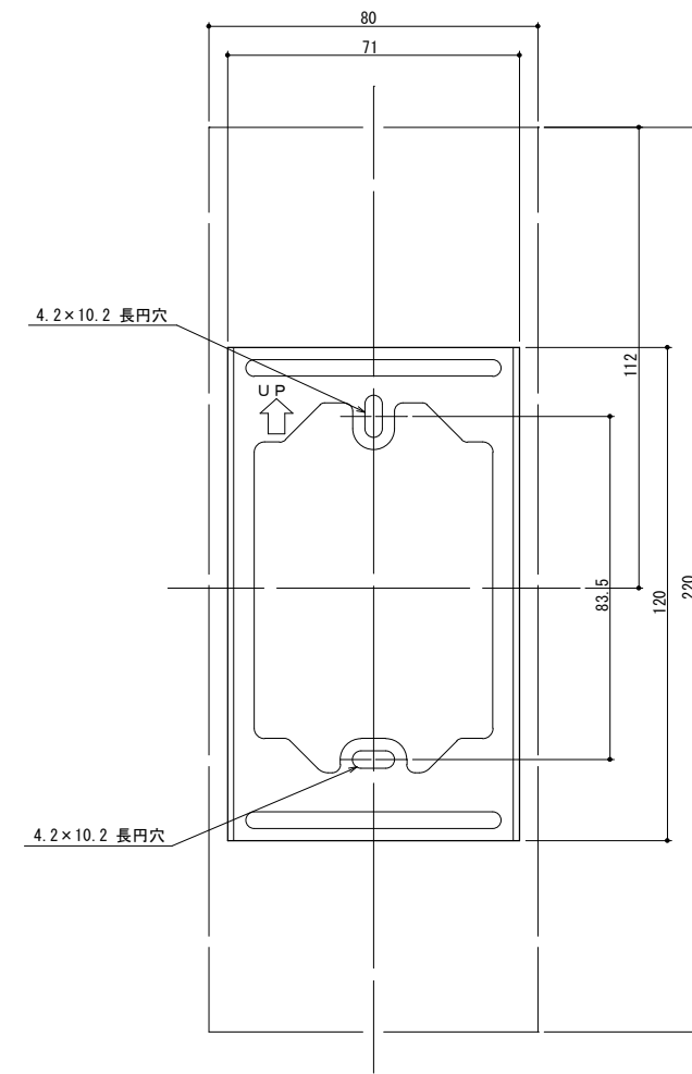
壁取付位置図 ※ 取付はM4ねじにて2箇所止め
