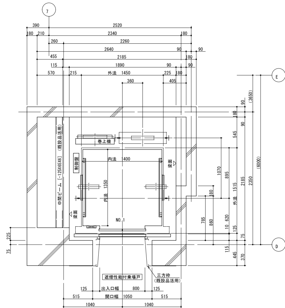
2階 昇降路平面図 (1 : 40)
