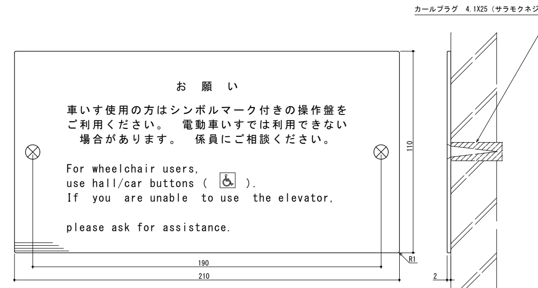
B1, 1~3階 車いす注意銘板 (乗場用) (1 : 2)
