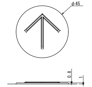
押しボタン意匠 (1 : 2)
