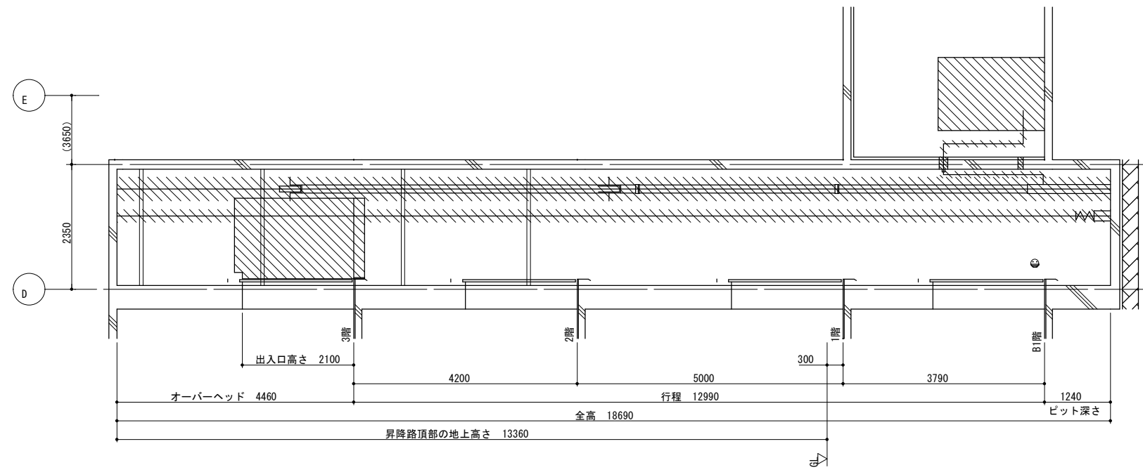
（撤去）昇降路断面図（1：100）
