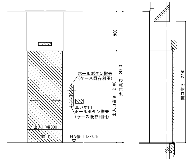
（撤去）1階 出入口正面及断面図（1：50）
