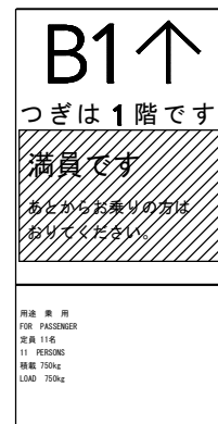
用途銘板及び表示部詳細図 (1 : 5)
