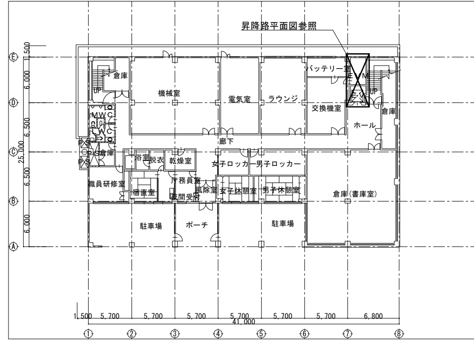
B1階平面図 S=1/500
