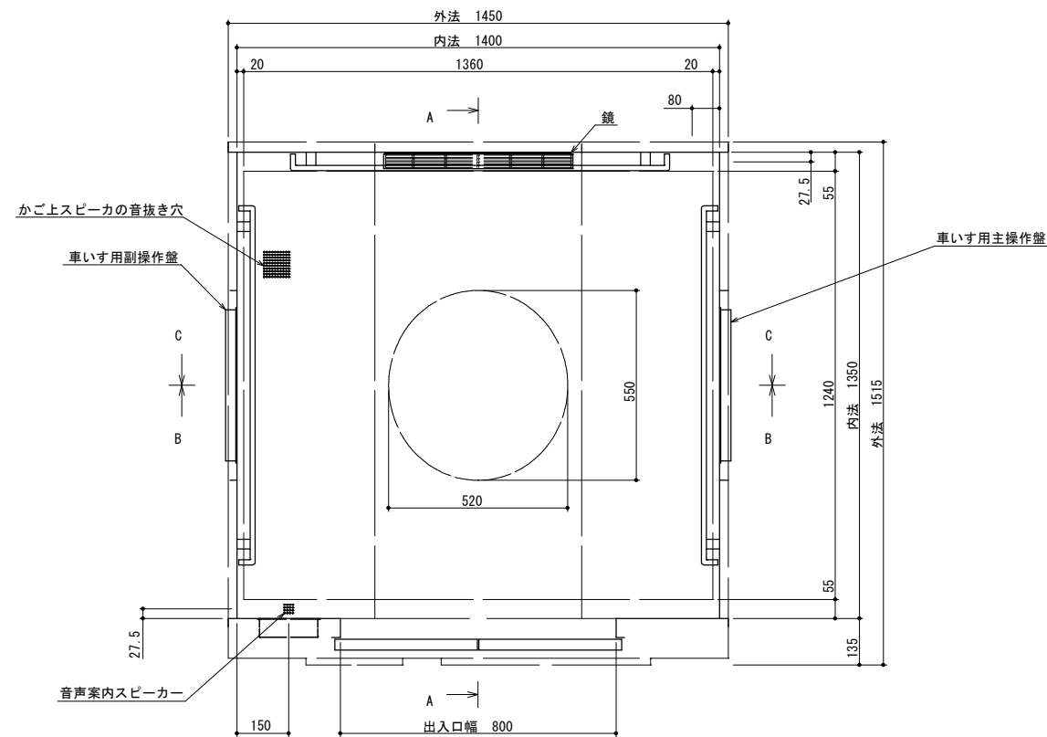
かご平面図 (1:20)
