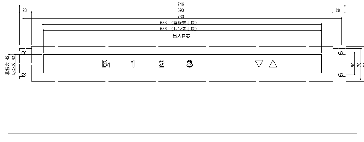
1階 インジケータ意匠図 (1:5)
