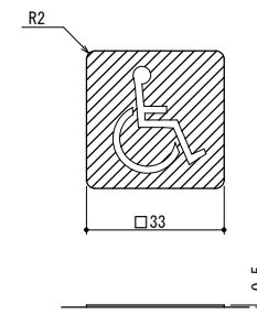
車いすマーク意匠 (1 : 2)
