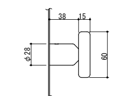
ハンドル取付部詳細 (1:5)
