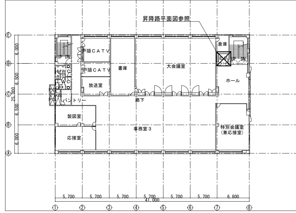
2階平面図 S=1/500
