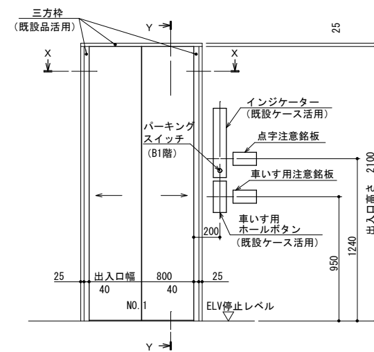
B1、2、3階 出入口正面図 (1:40)
