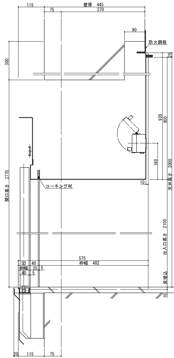
断面図 [断面YY] (1:10)
