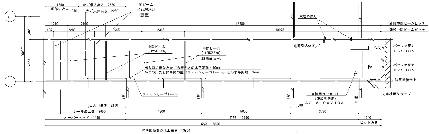
昇降路断面図 (1:100)
