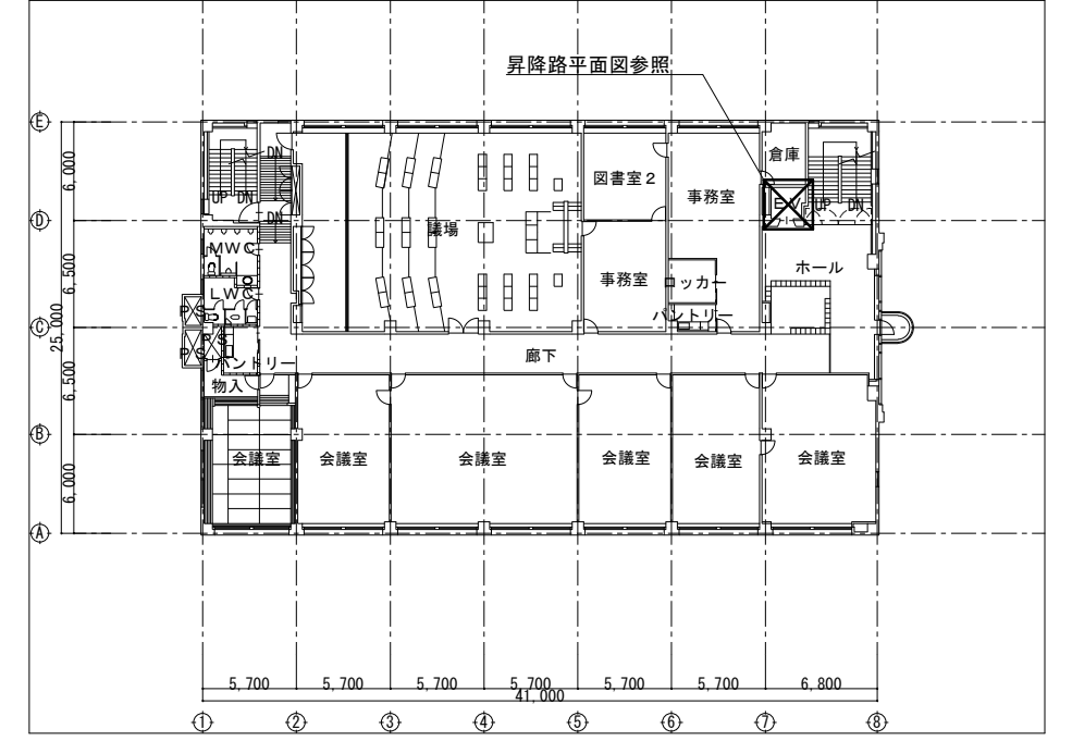
3階平面図 S=1/500
