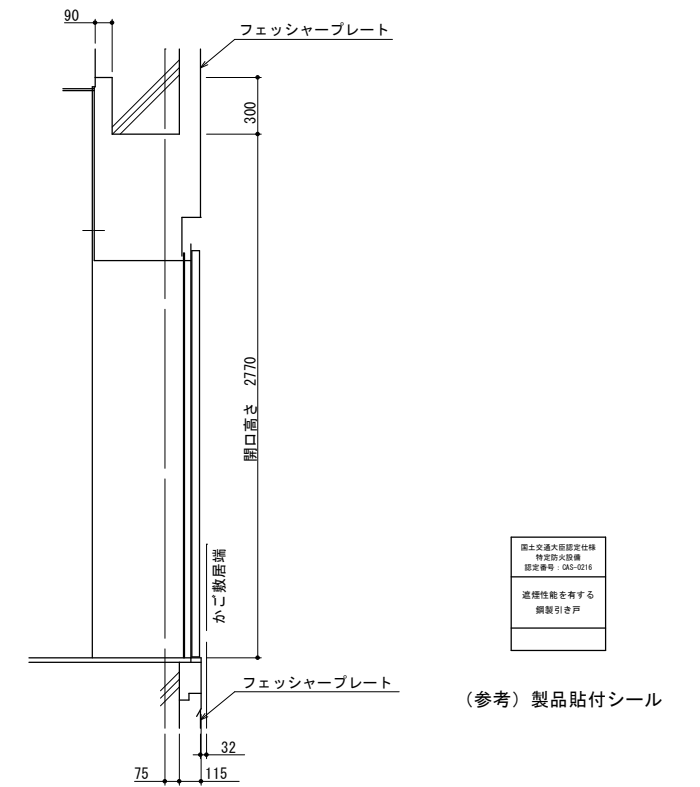
1階 出入口正面及断面図 (1:40)
