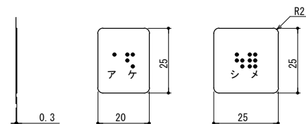
点字銘板意匠 (1 : 2) 点字下部の数字、片仮名は参考
