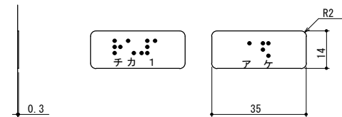
点字銘板意匠 (1 : 2) 点字下部の数字, 片仮名は参考
