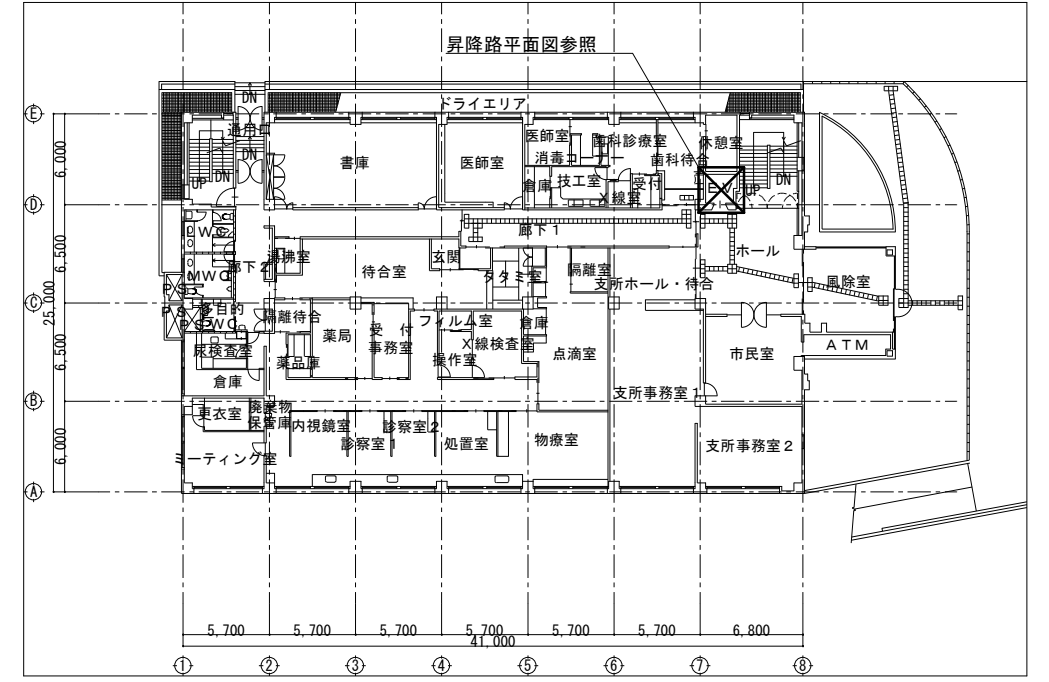
1階平面図 S=1/500
