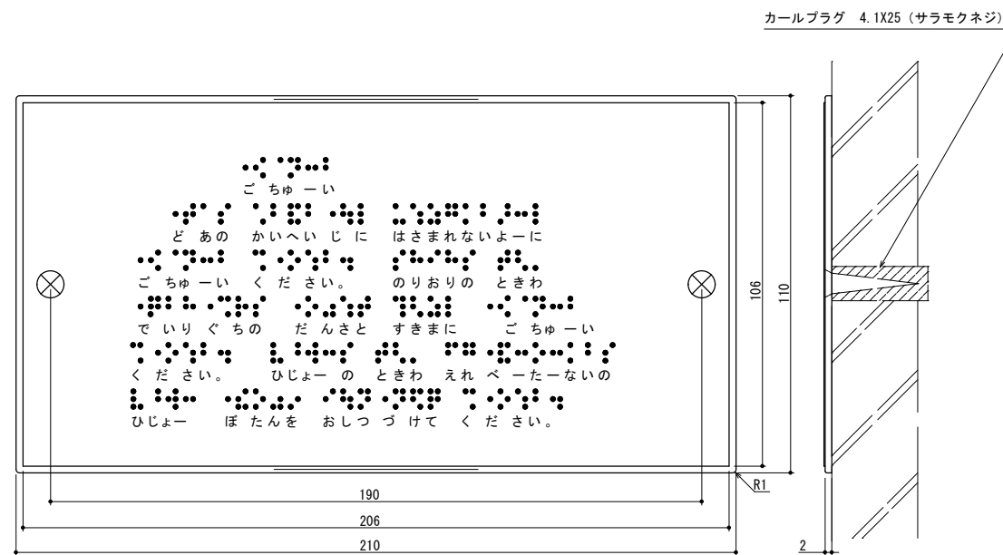
B1, 1~3階 点字注意銘板 (乗場用) (1 : 2)
