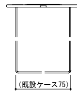
B1, 1~3階 車いす用ホールボタン意匠図 (1 : 5)
