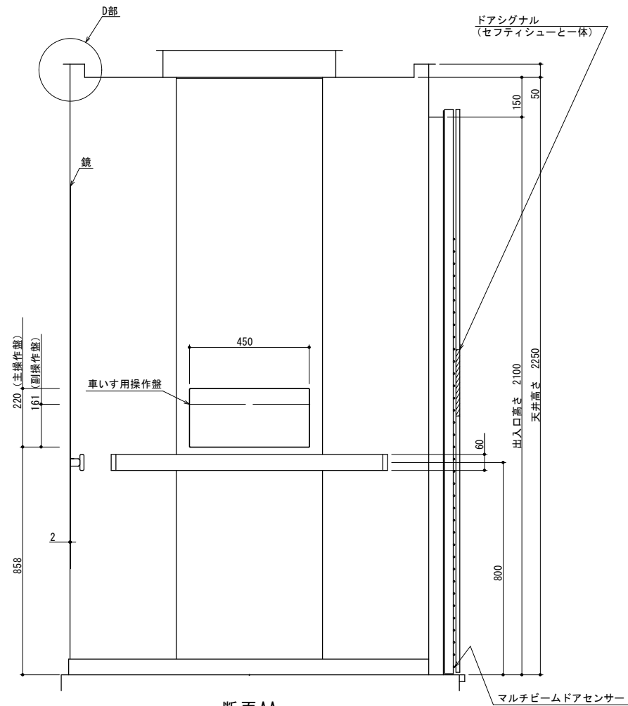
断面AA
