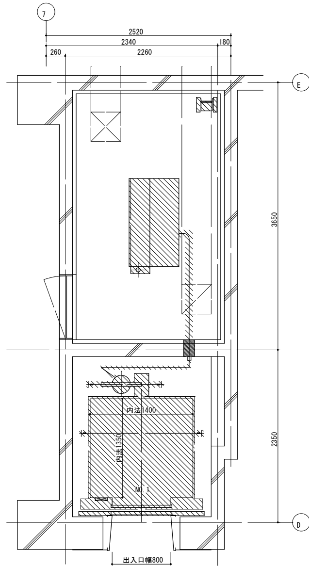
（撤去）昇降路平面図（1：50）
