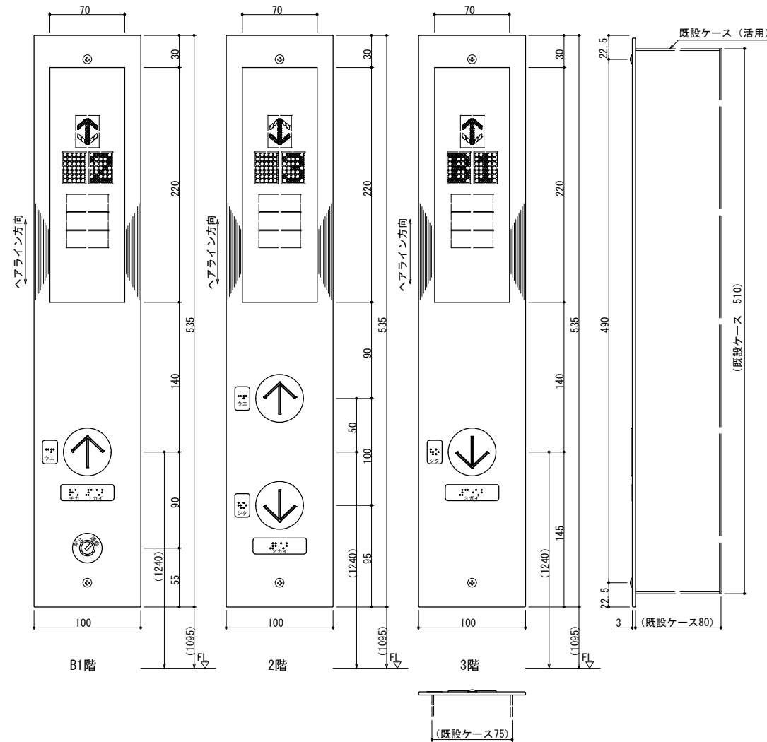
B1、2、3階 インジケータ意匠図 (1:5)
