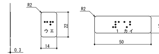
点字銘板意匠 (1 : 2) 点字下部の数字、片仮名は参考
