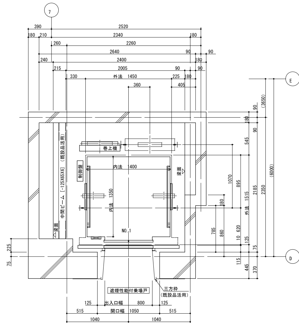
3階 昇降路平面図 (1 : 40)
