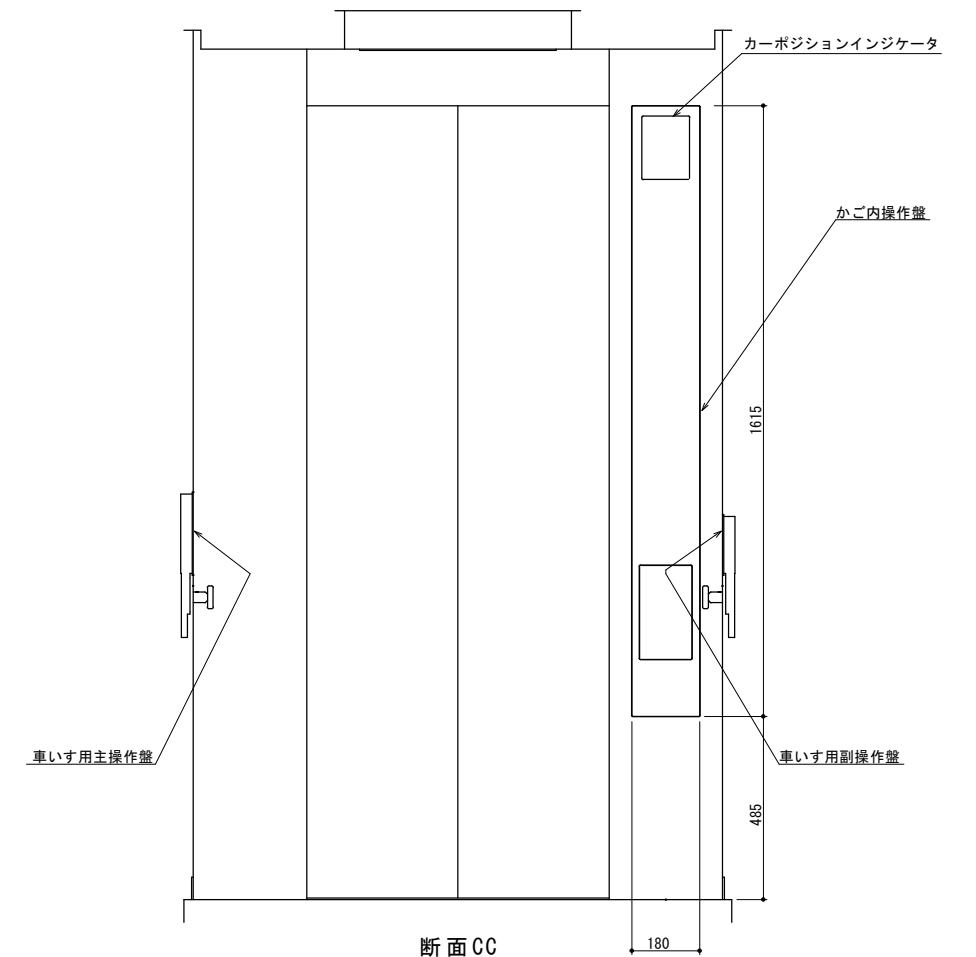
断面CC
