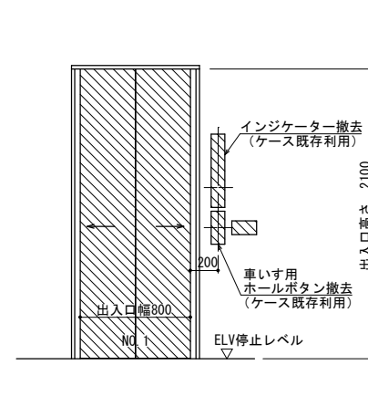
（撤去）B1、2、3階 出入口正面及断面図（1：50）
