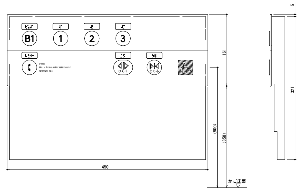
副操作盤 (1 : 5)
