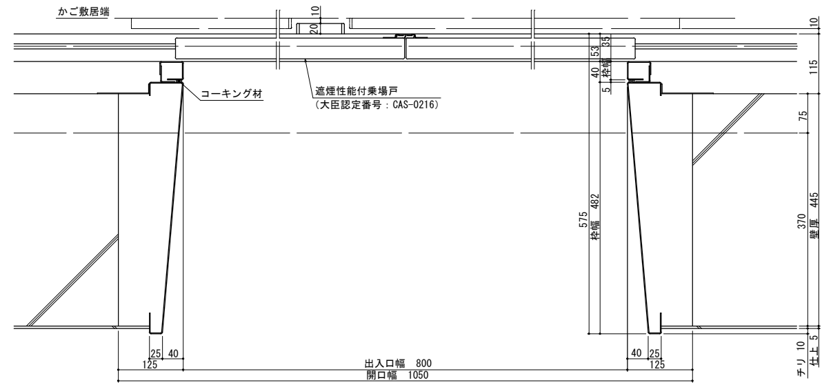
平面図 [断面XX] (1:10)
