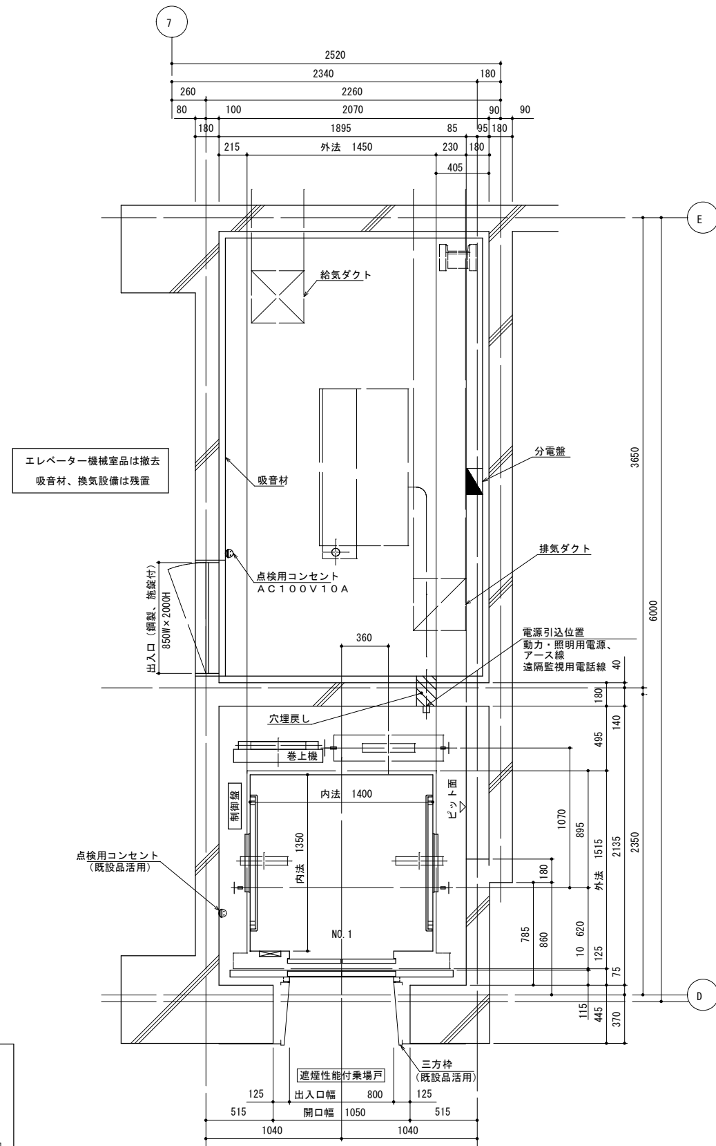
B1、1階 昇降路平面図 (1 : 40)
