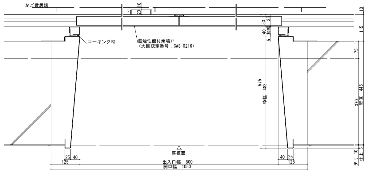
平面図 [断面XX] (1:10)
