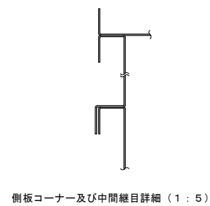
側板コーナー及び中間継目詳細 (1:5)
