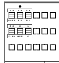
下部スイッチボックス内 (1 : 5)
