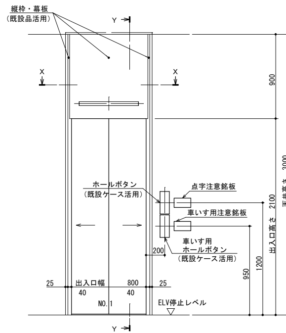
1階 出入口正面及断面図 (1:40)
