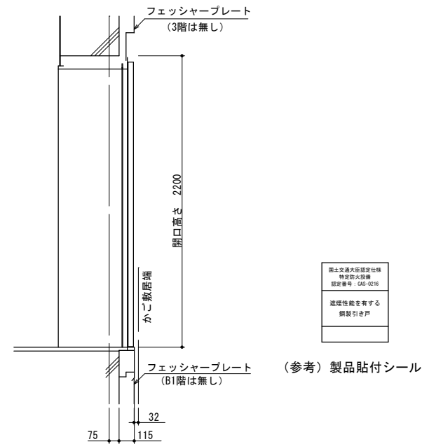
B1、2、3階 出入口正面及断面図 (1:40)
