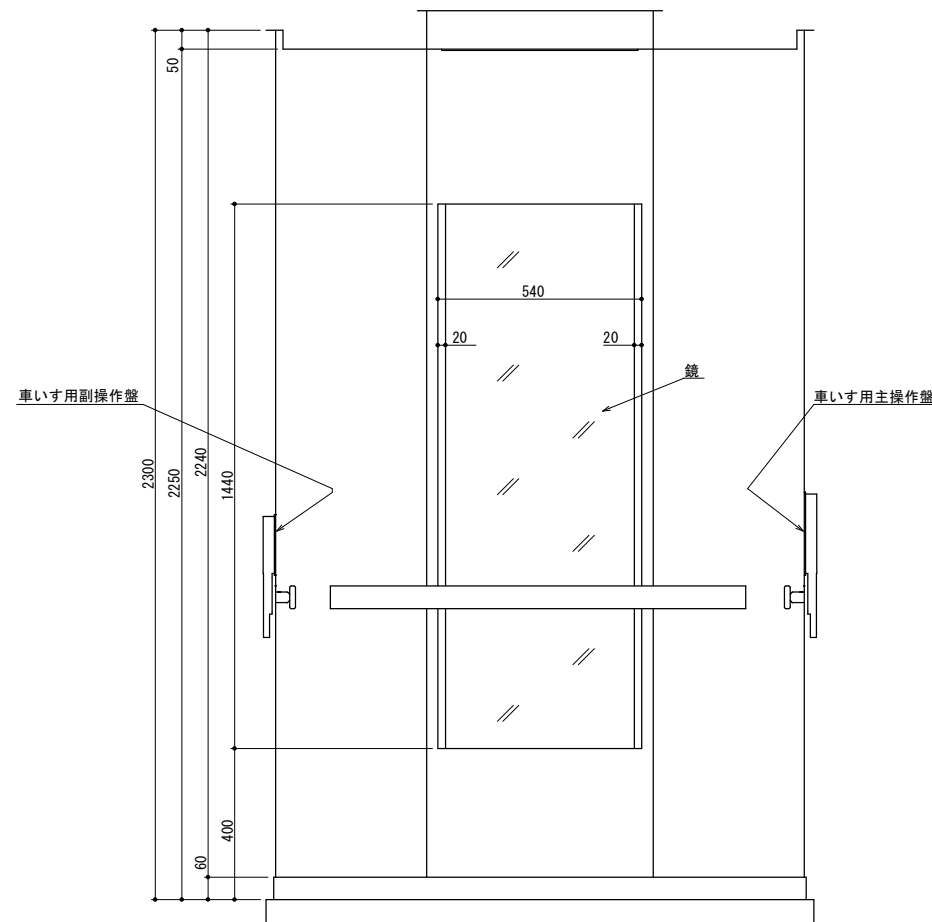
断面BB
