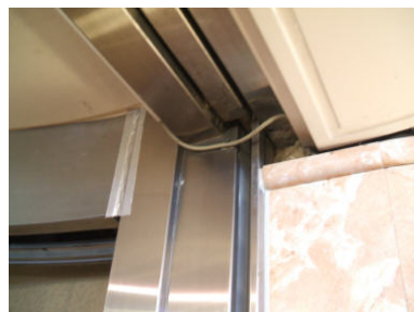
配線による閉鎖障害
