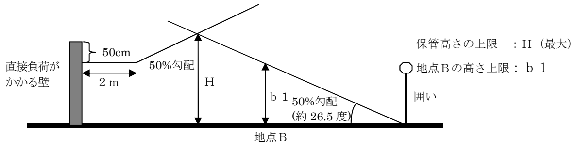
図 保管高さの基準例（屋外に容器を用いずに保管する場合）
