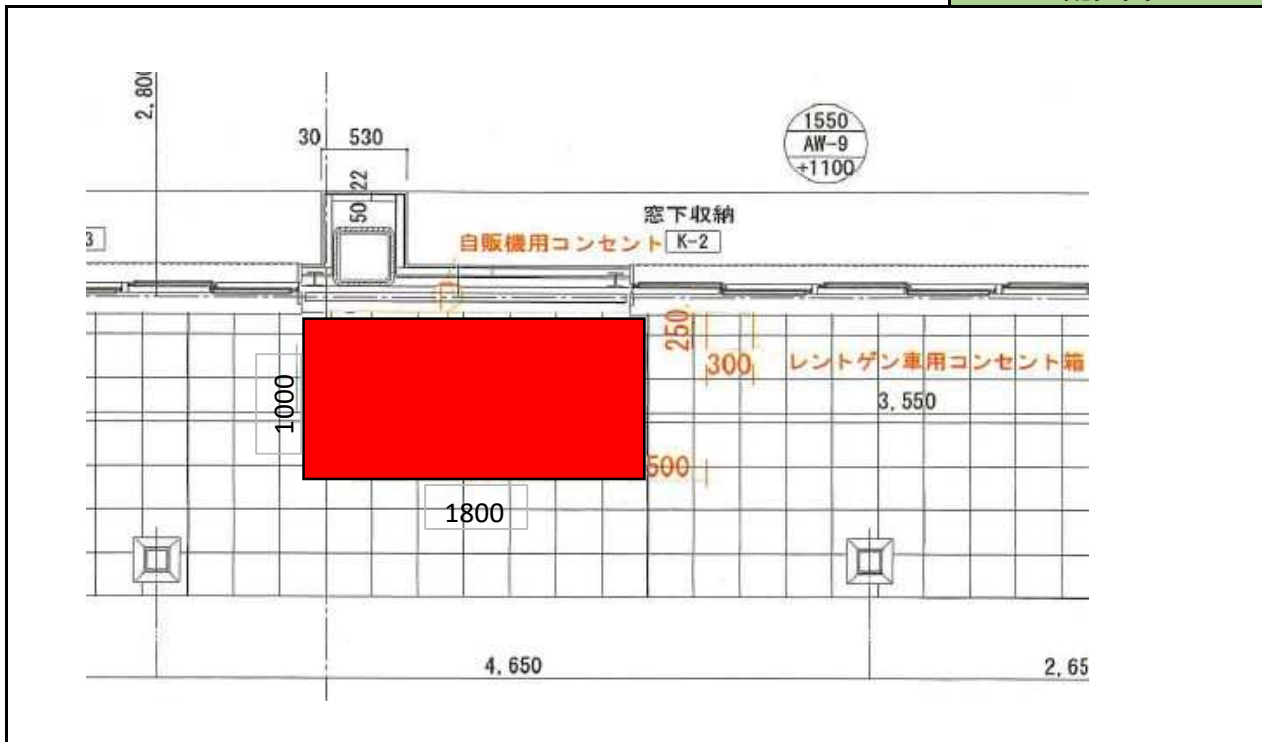
配置図
