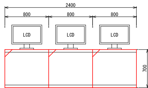
正面図
