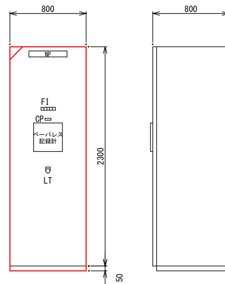
正面図
