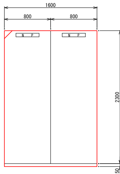
正面图
