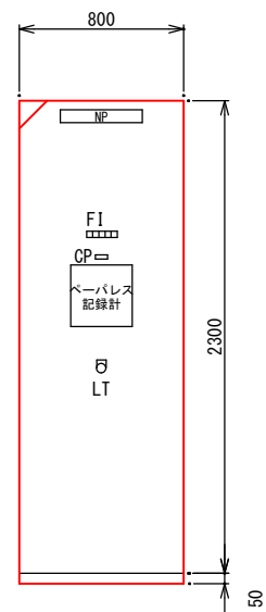
正面図
