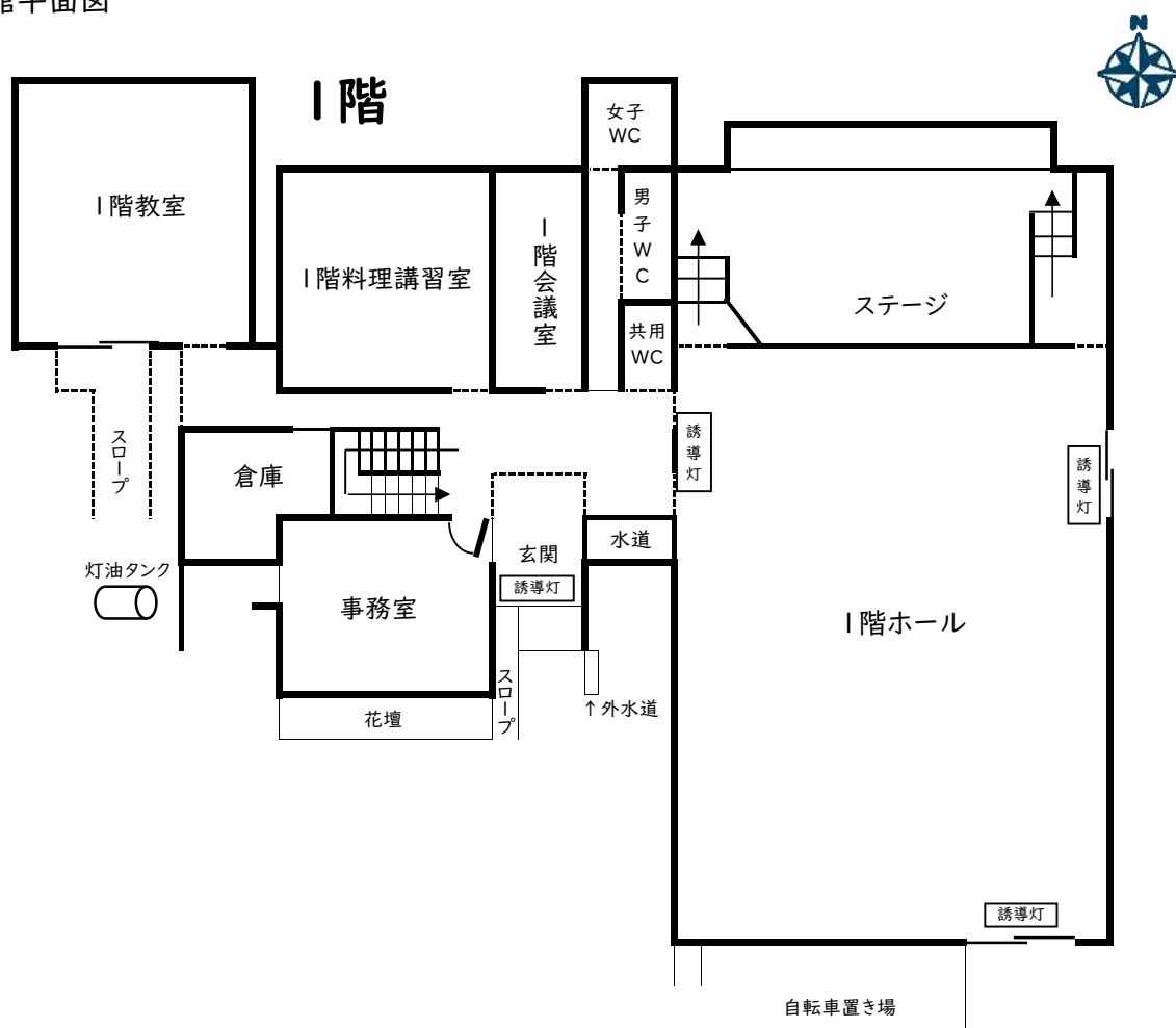
本館平面図
