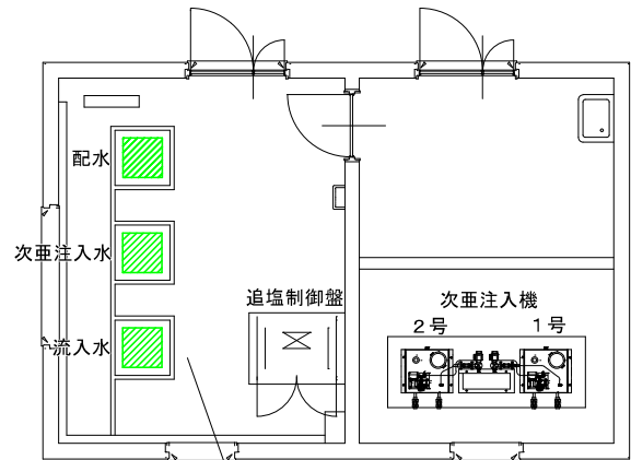
上野配水池 次亜室 平面図 S=1:100
