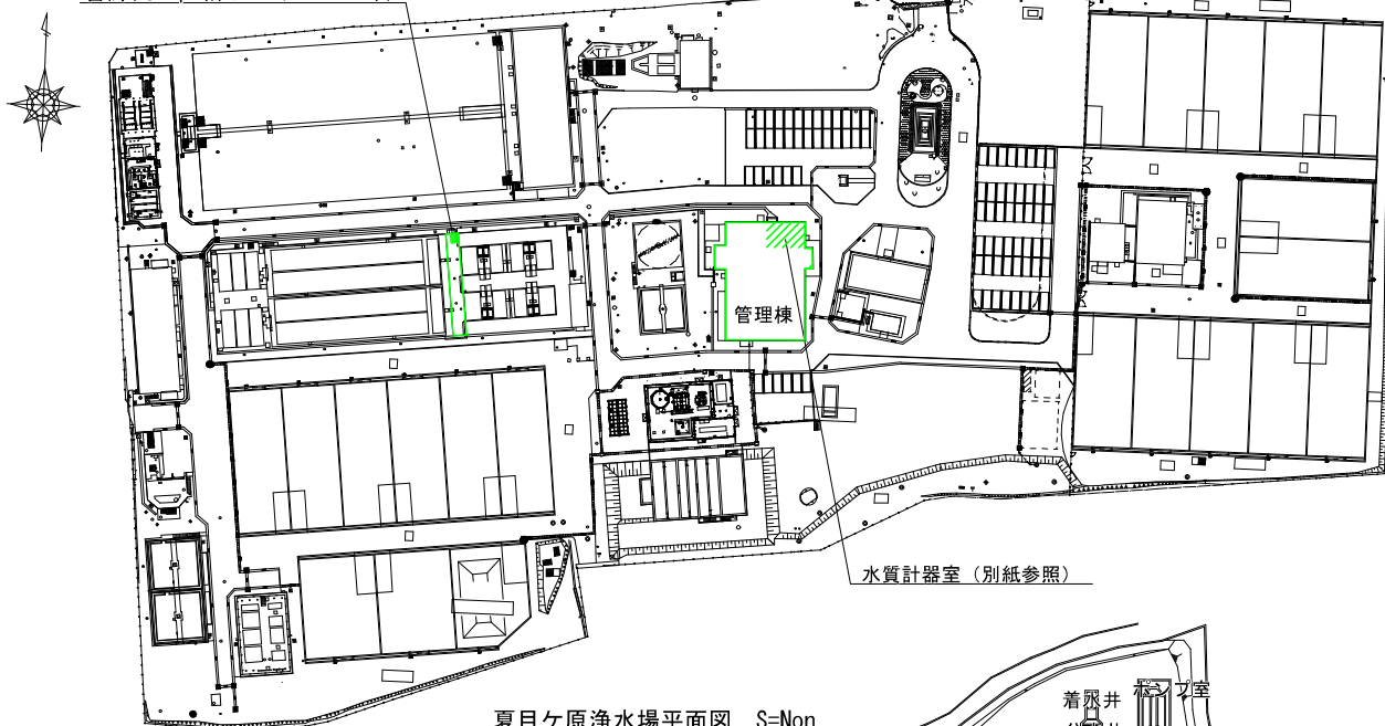
夏目ヶ原浄水場平面図 S=Non
