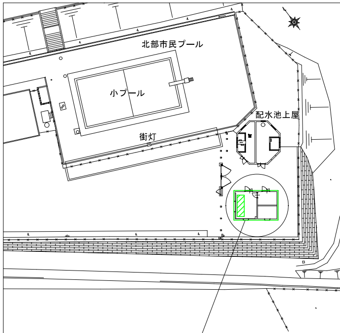
上野配水池 次亜室 平面図 参照
