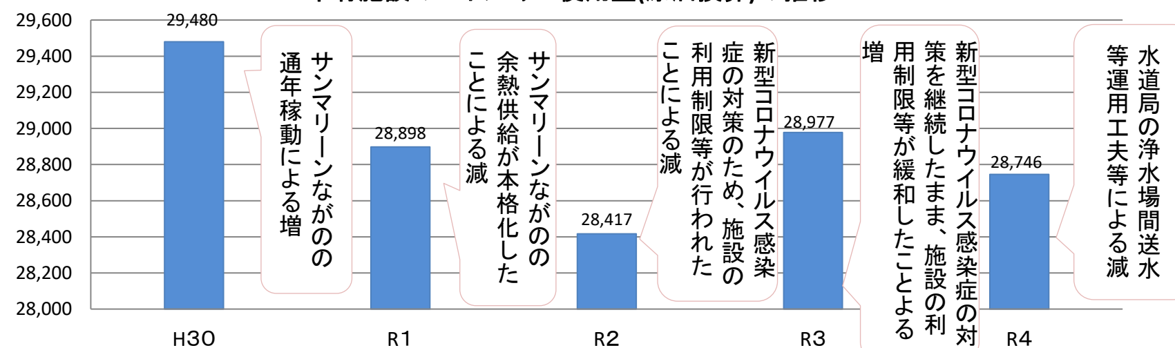
(kℓ) 市有施設のエネルギー使用量(原油換算)の推移
