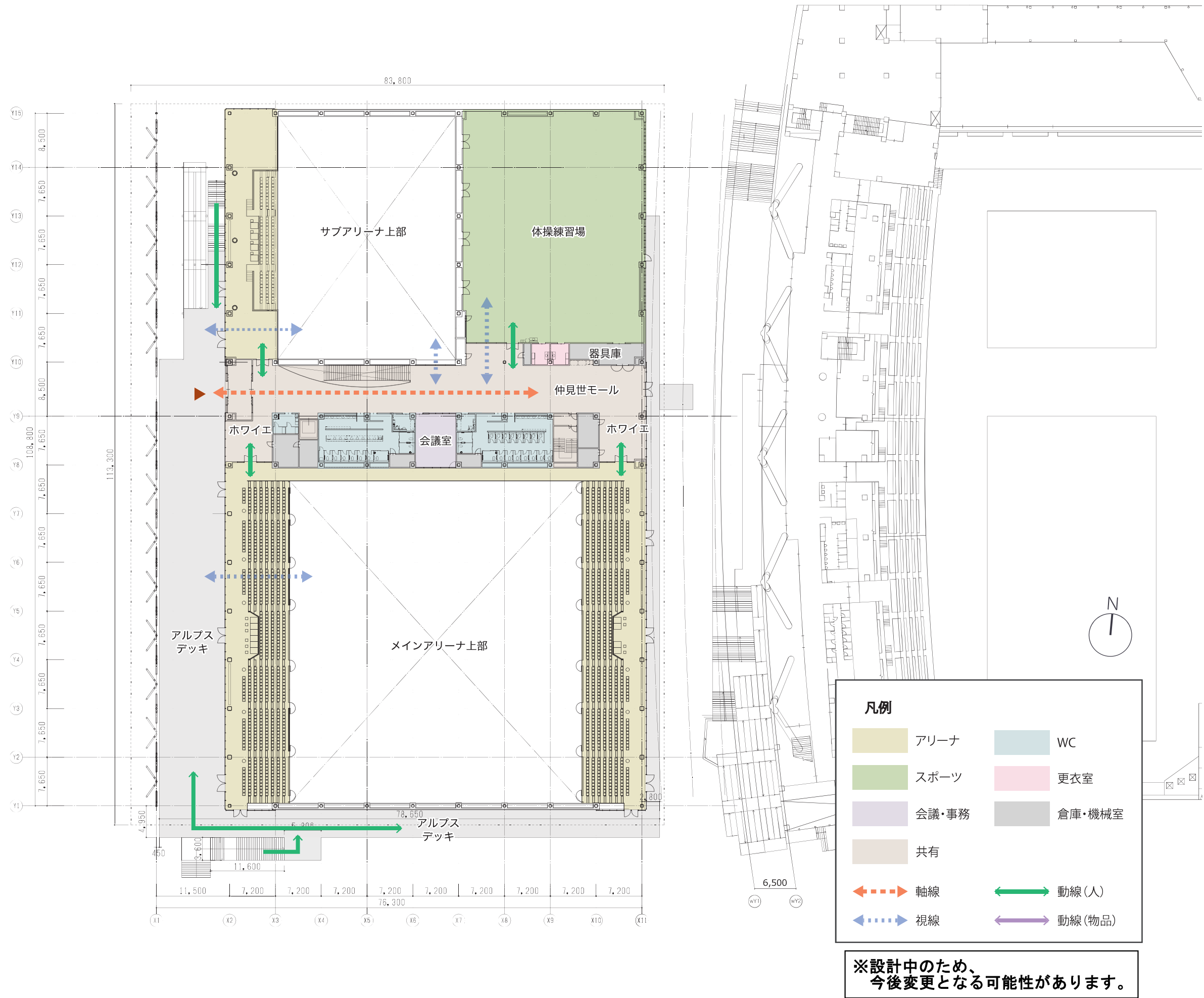
長野運動公園総合体育館 2階 平面図
