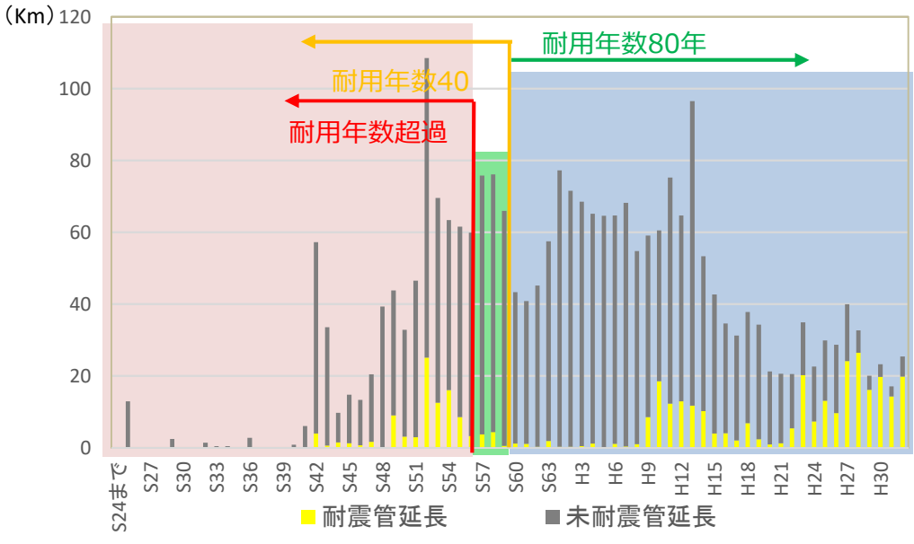
図7 管路の年度別敷設状況
