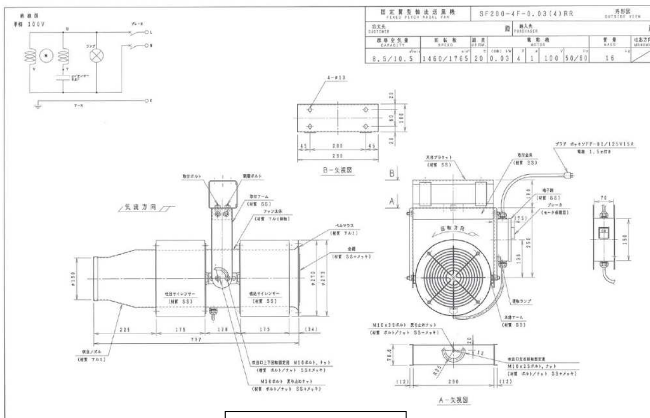
デリベントファン参考図
