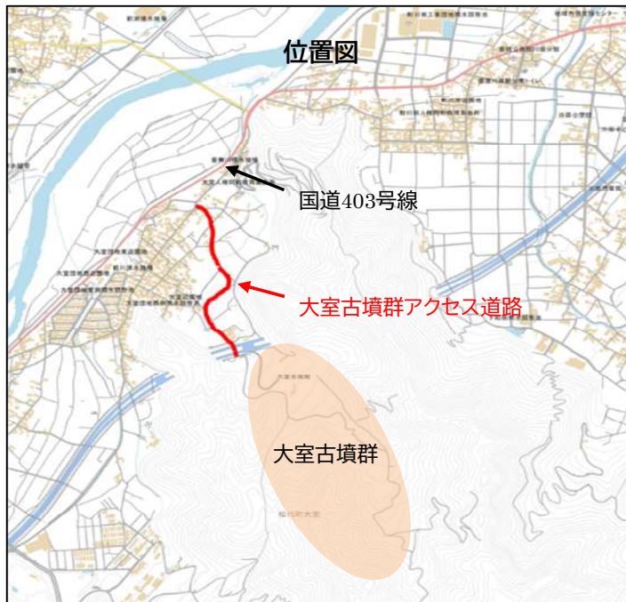
大室古墳群アクセス道路 詳細設計図(全体図)
