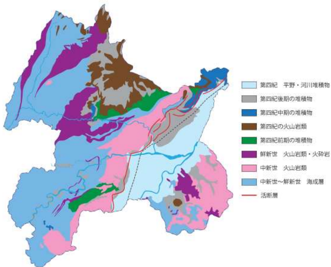
長野市地質図
