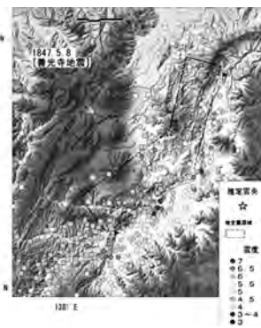
地震の震央は野尻湖の東側と考えられています(松浦説)。「弘化善光寺地震の長野盆地での震度分布図」(内閣府中央防災会議資料より 松浦氏作図)
