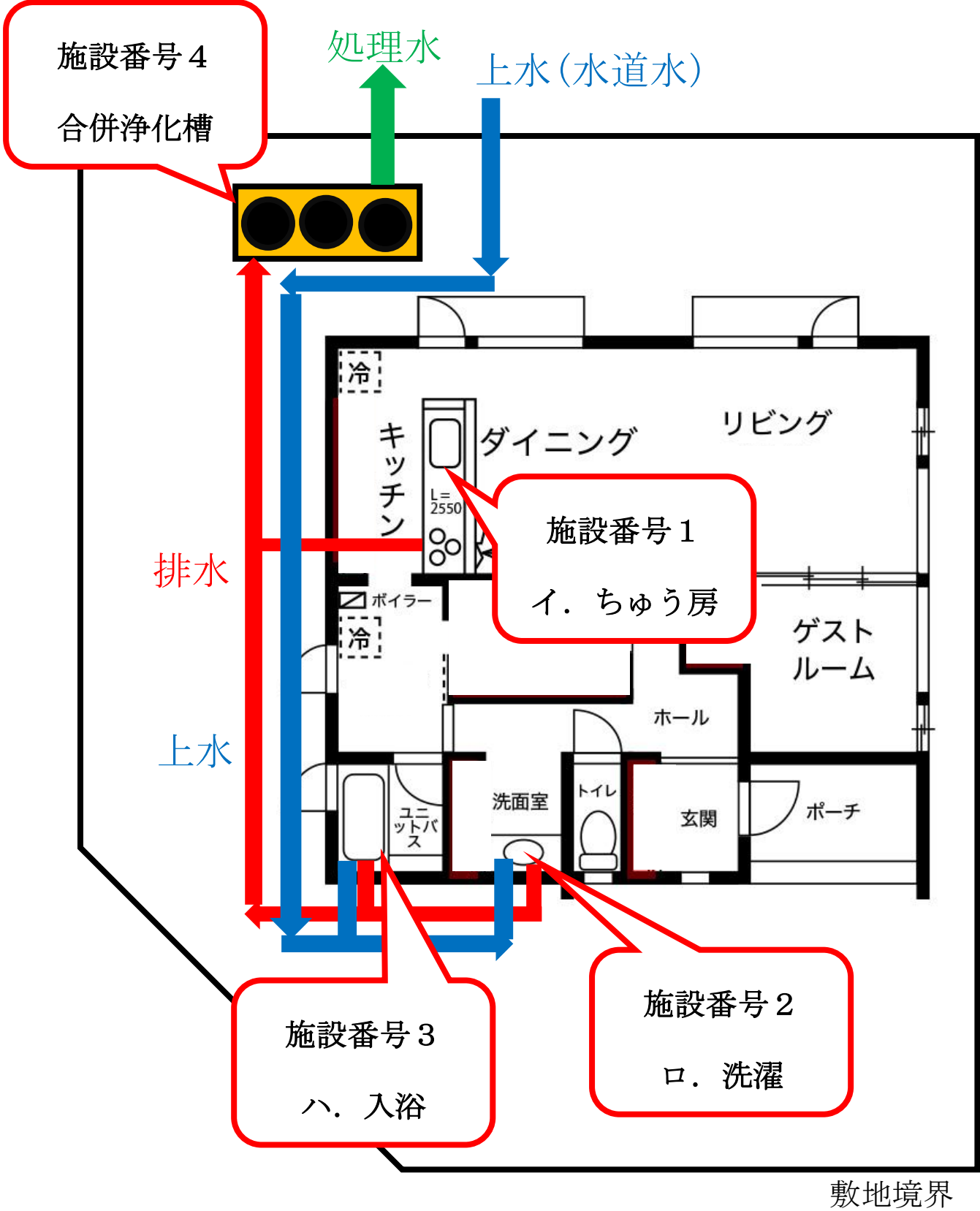
別図(配置図)(用水排水の系統図)
