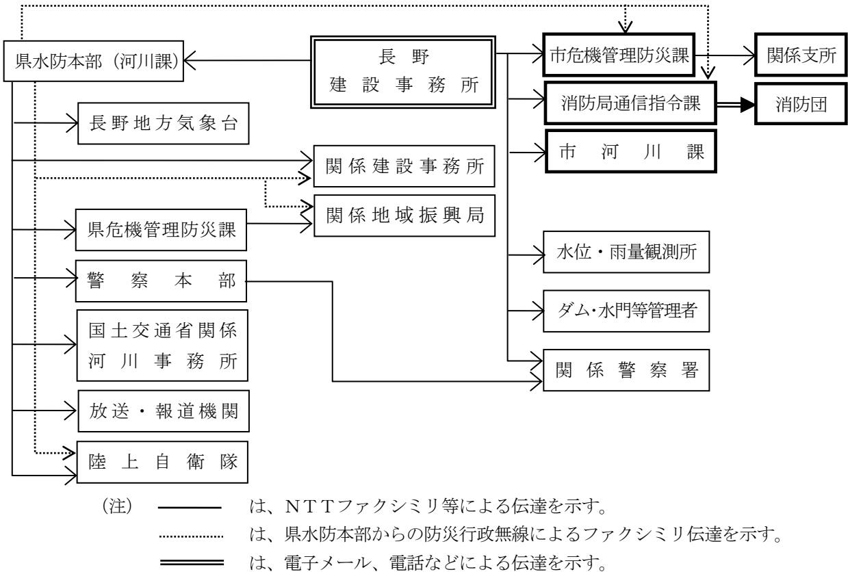
〈水防警報の伝達系統図〉
