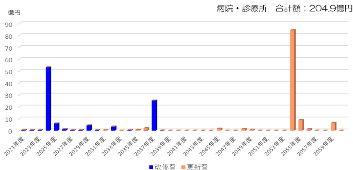
図9 自然体による今後40年間の改修・更新費用推計
