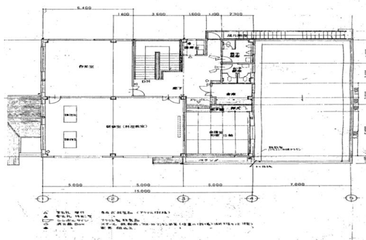
2階見取図
