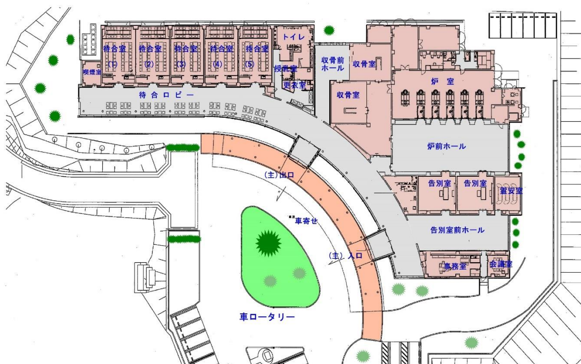
大峰新斎場の主な諸室
