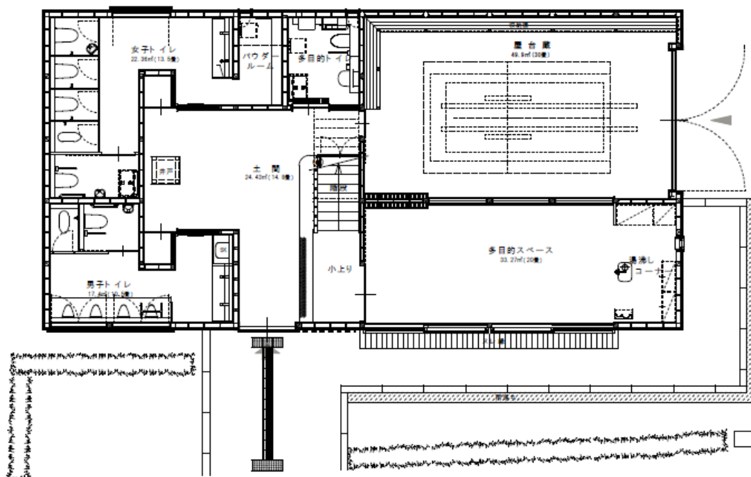
東町会館 1 階平面図
