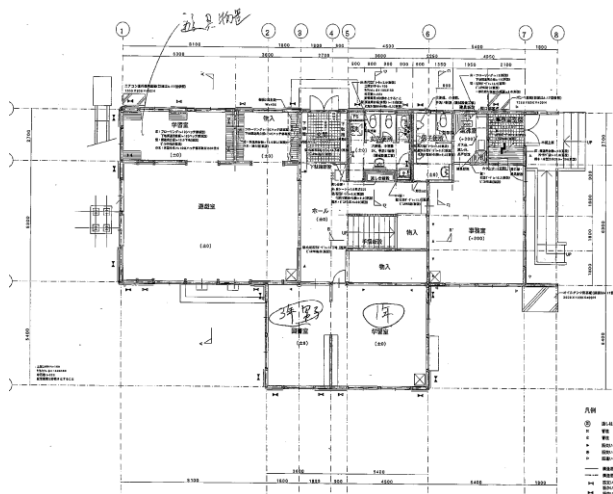
1階見取り図
