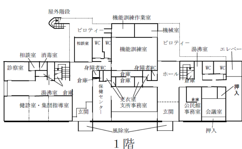
安茂里公民館 平面図
