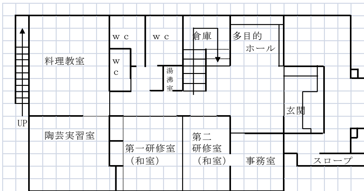
1 階
