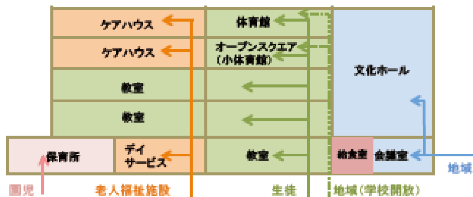
<立面図>
