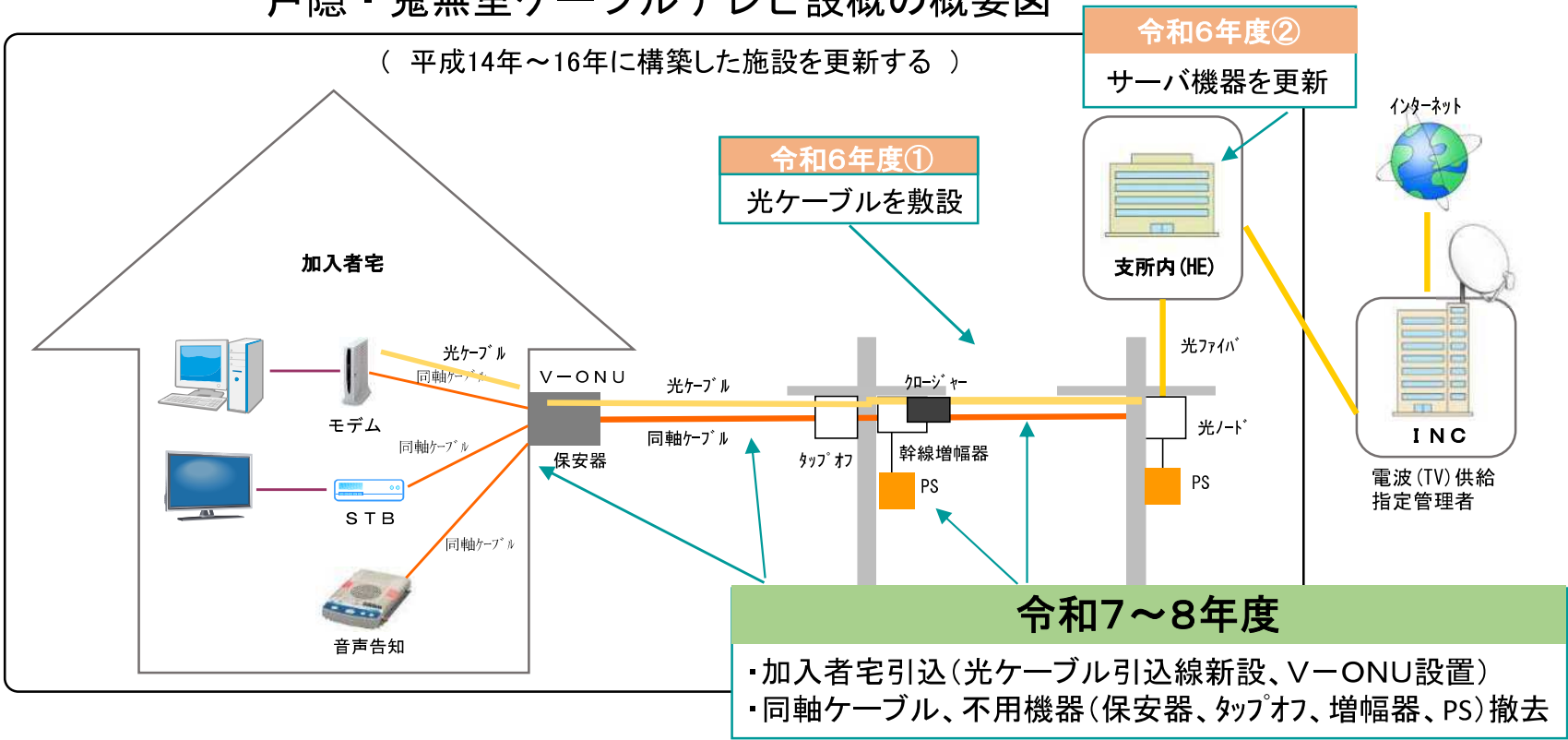
戸隠・鬼無里ケーブルテレビ設概の概要図
