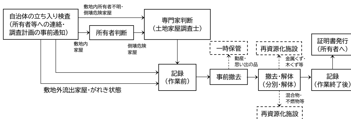
図3-9 損壊家屋等の撤去到に係る作業・処理フロー
