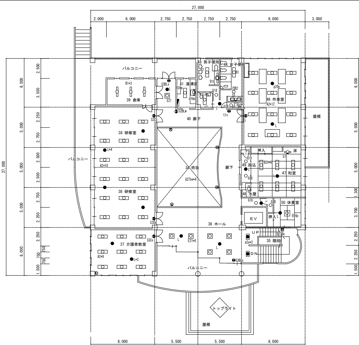
2階平面図 1 : 200
