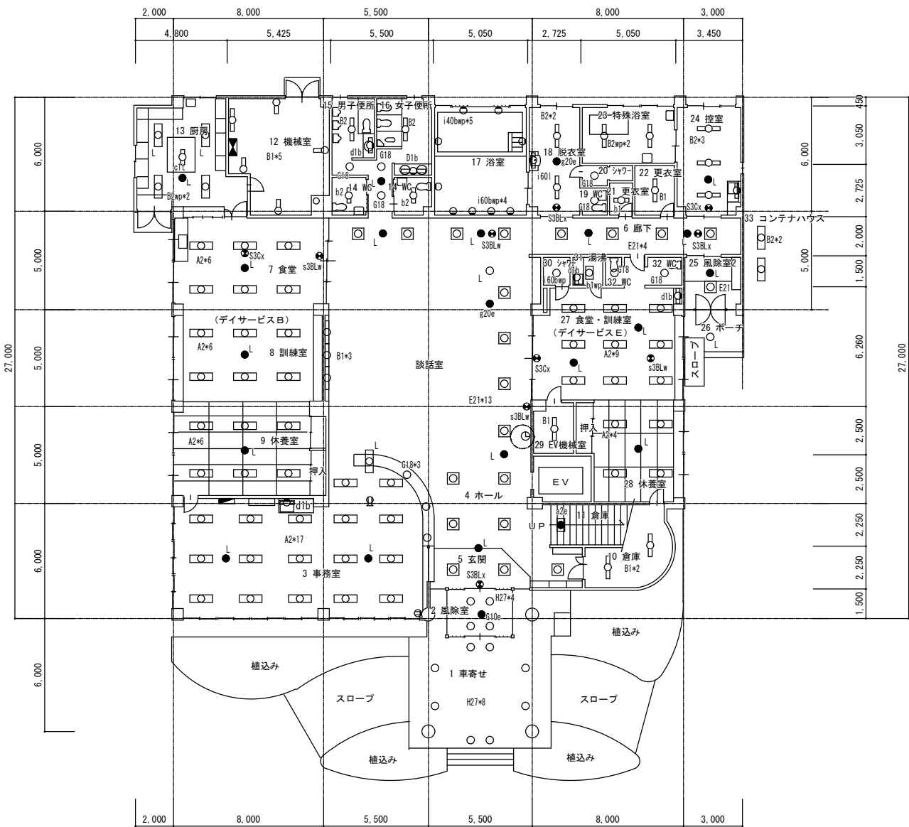
1階平面図 1 : 200
