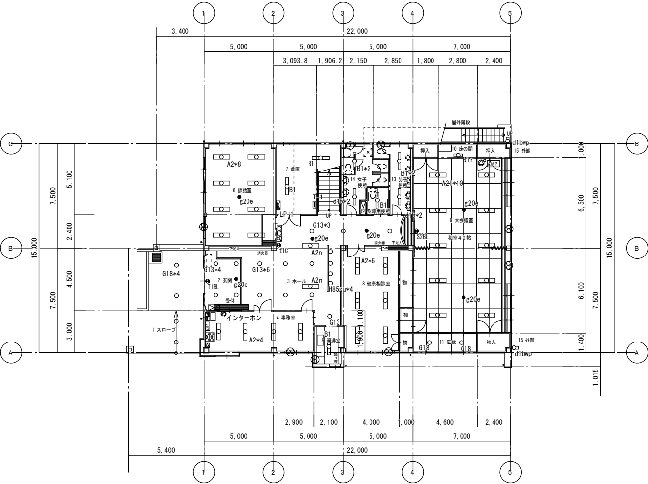
1階平面図 1/200
