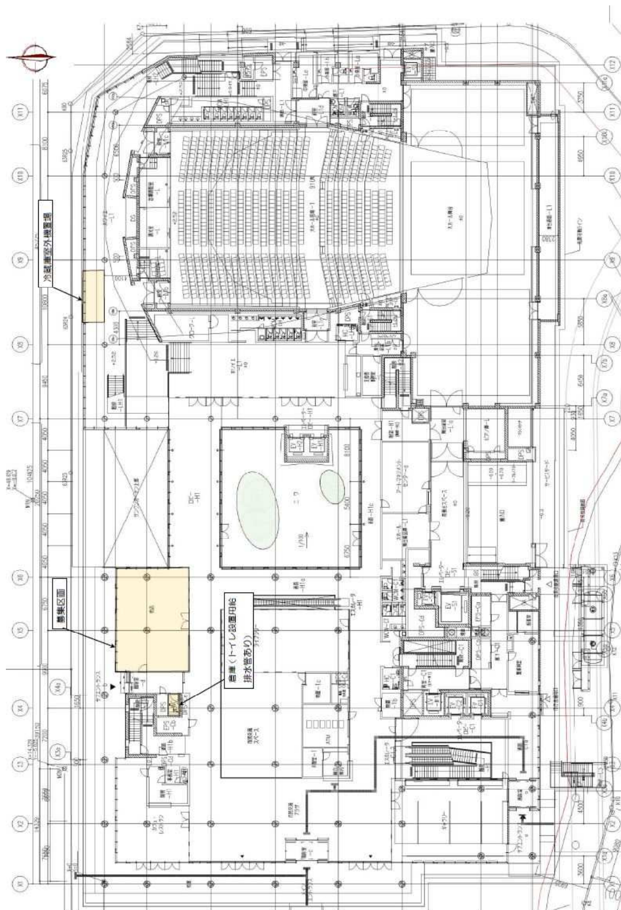
長野市第一庁舎 1 階及び長野市芸術館 図面
