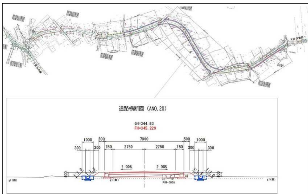
道路設計図
