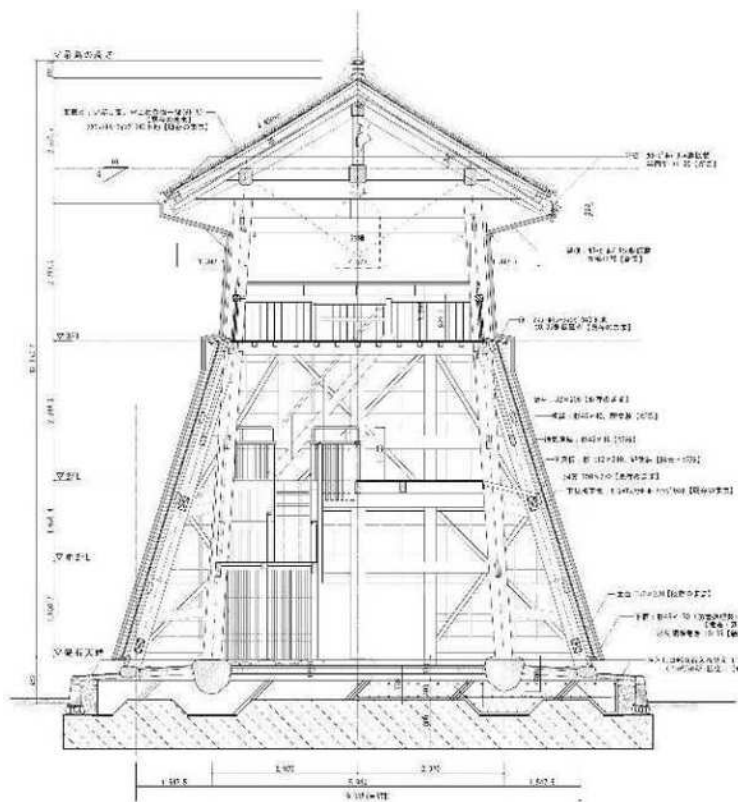
設計図（梁間方向）
