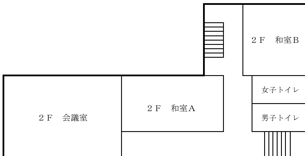
2 階
