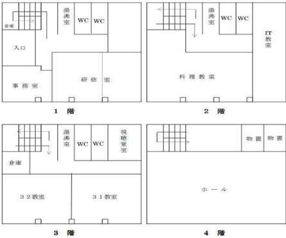
中部公民館 本館 平面図
