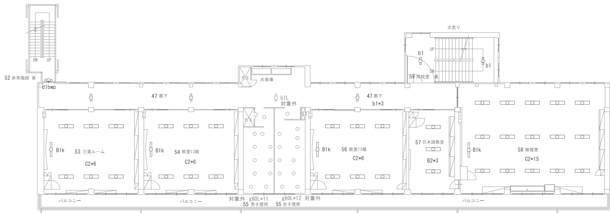
2階平面図 東
