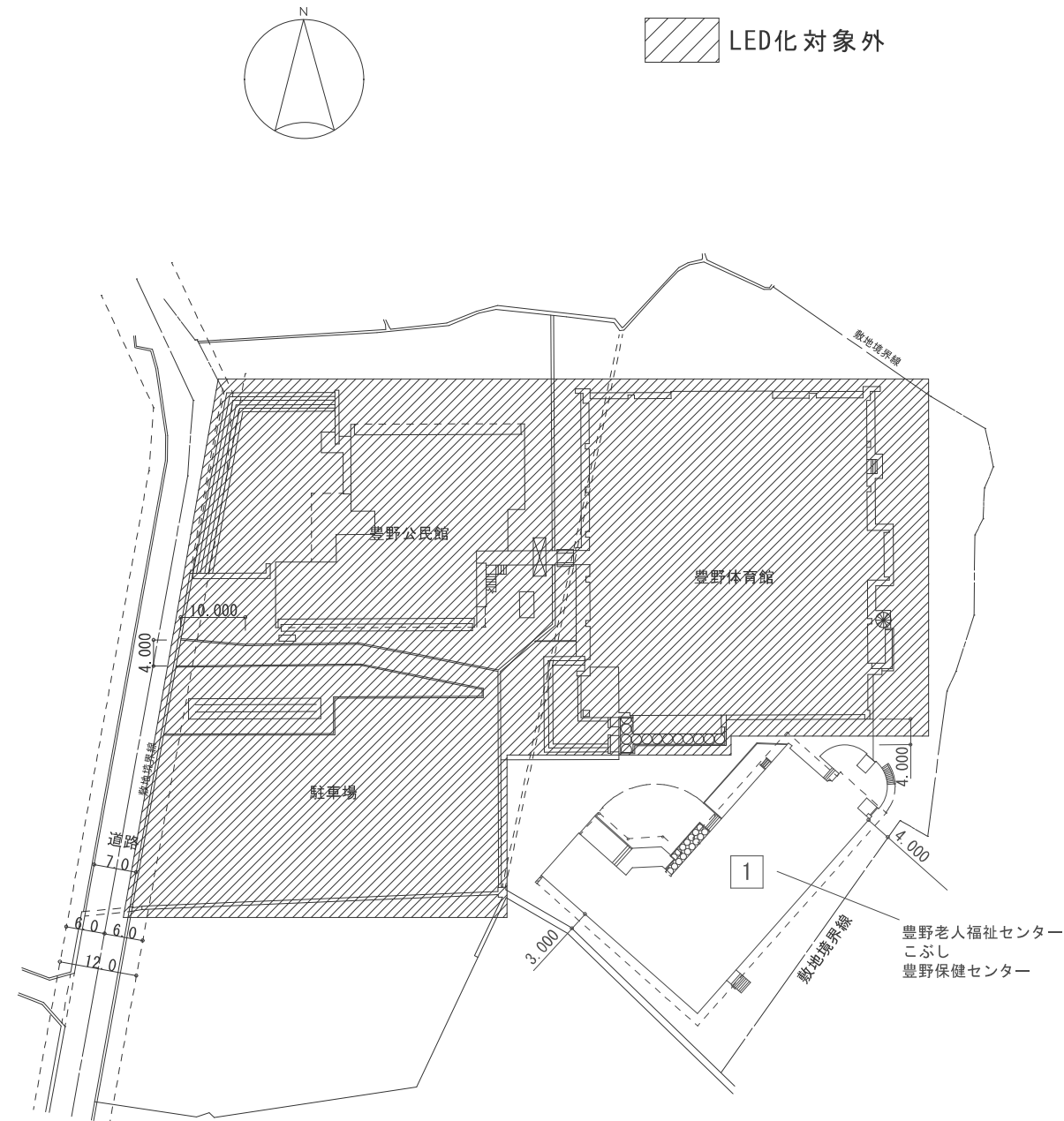
配置図
