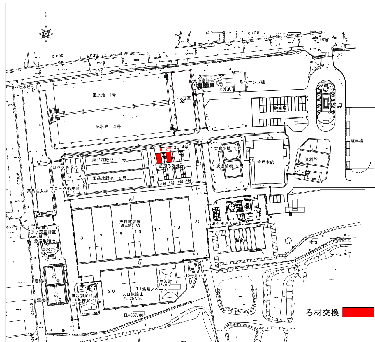
犀川浄水場平面図
