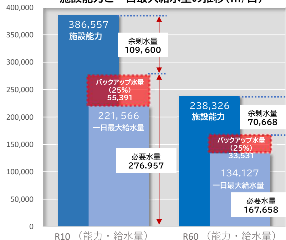
施設能力と一日最大給水量の推移( \text{m}^3/\text{日} )
