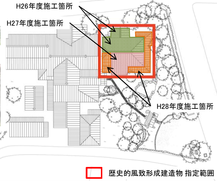
武井旅館 H28年度施工箇所 (主屋 西面屋根、下屋庇、外壁)
