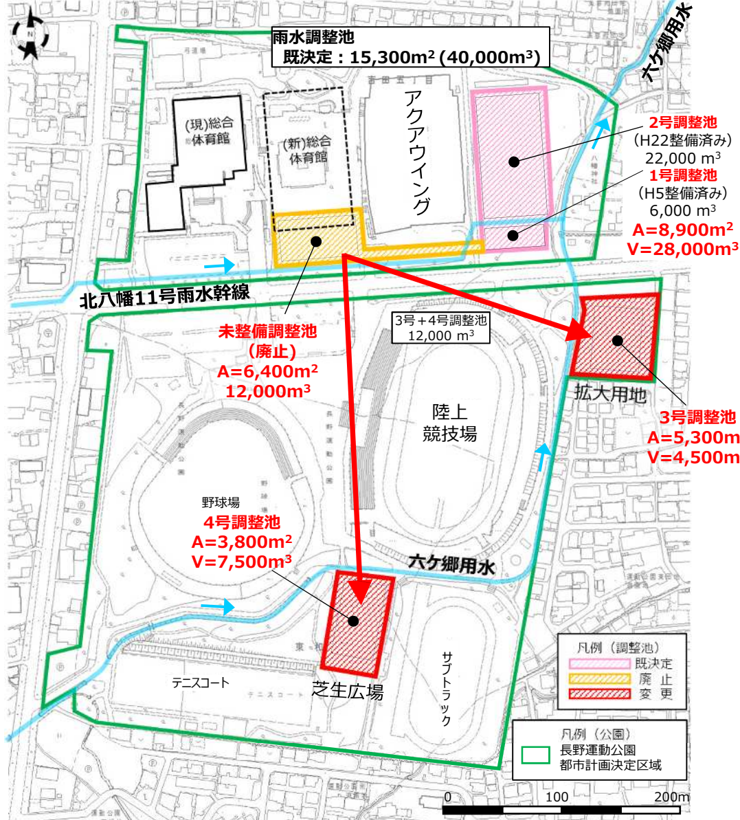
運動公園調整池 計画図
