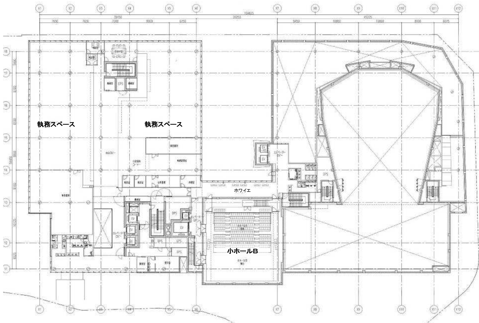
3階平面図
