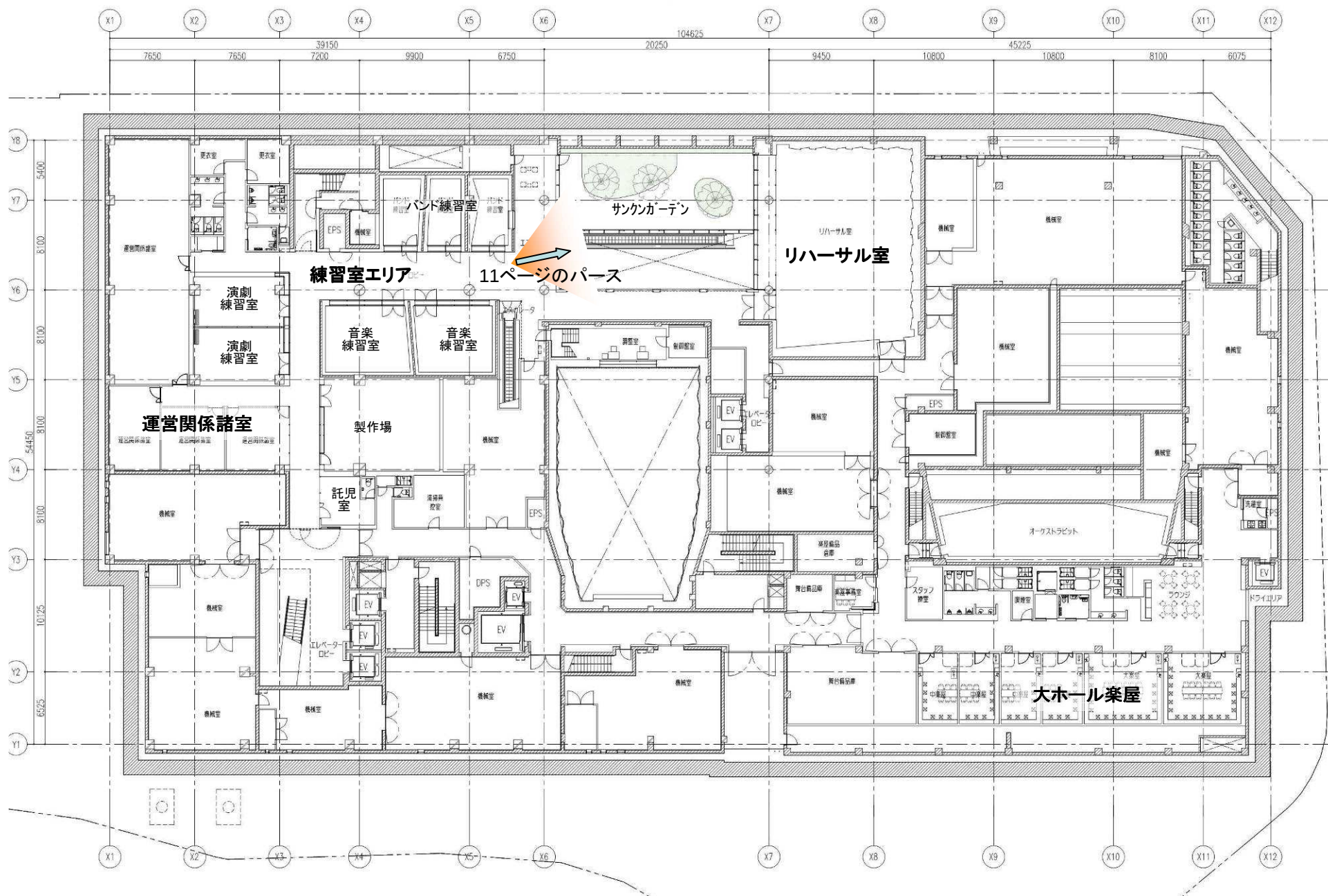
地下1階平面図
