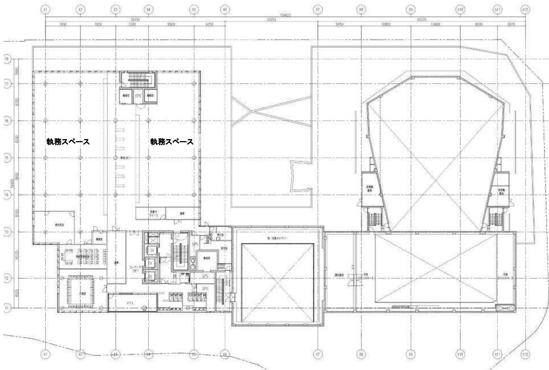
4階平面図
