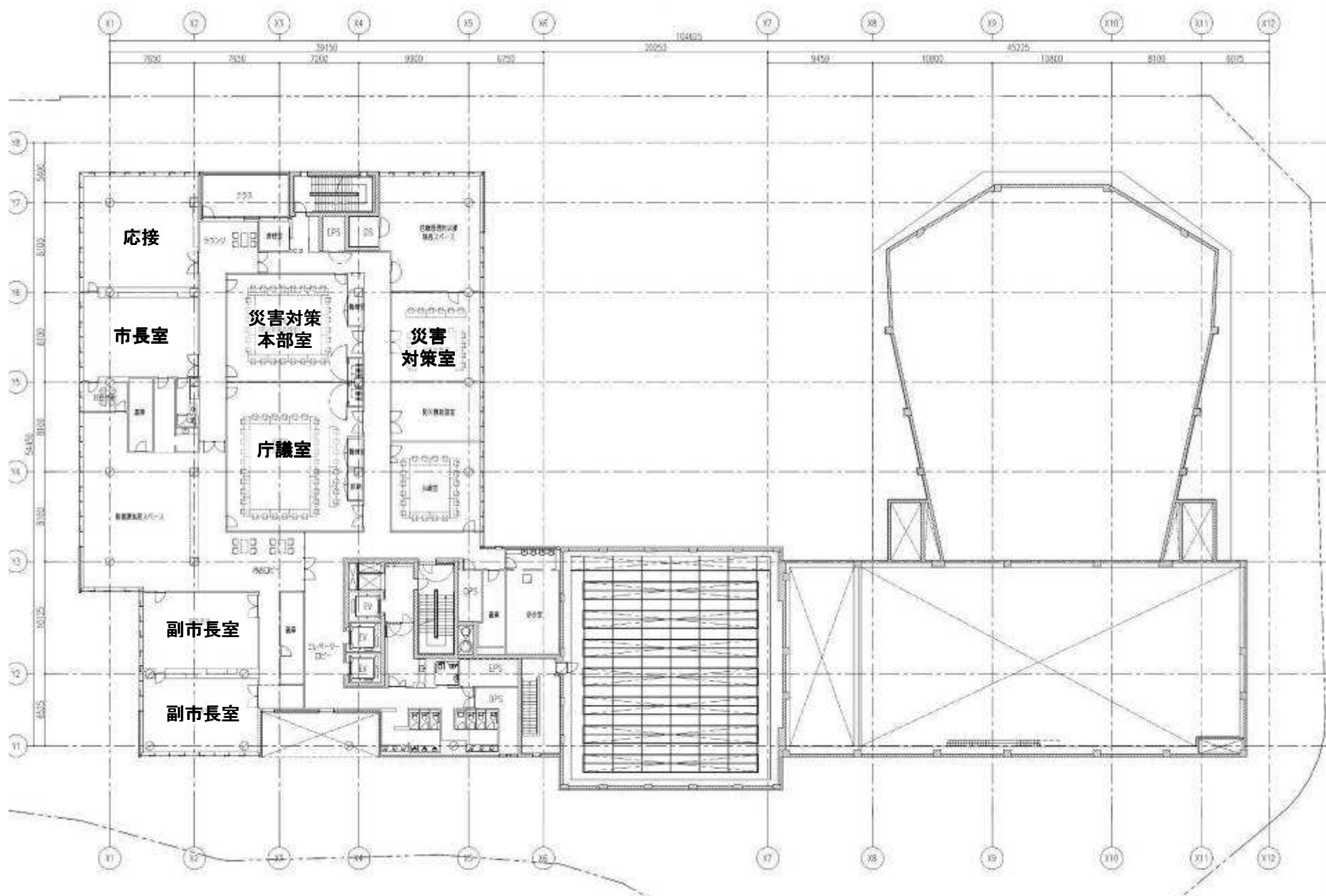
5階平面図
