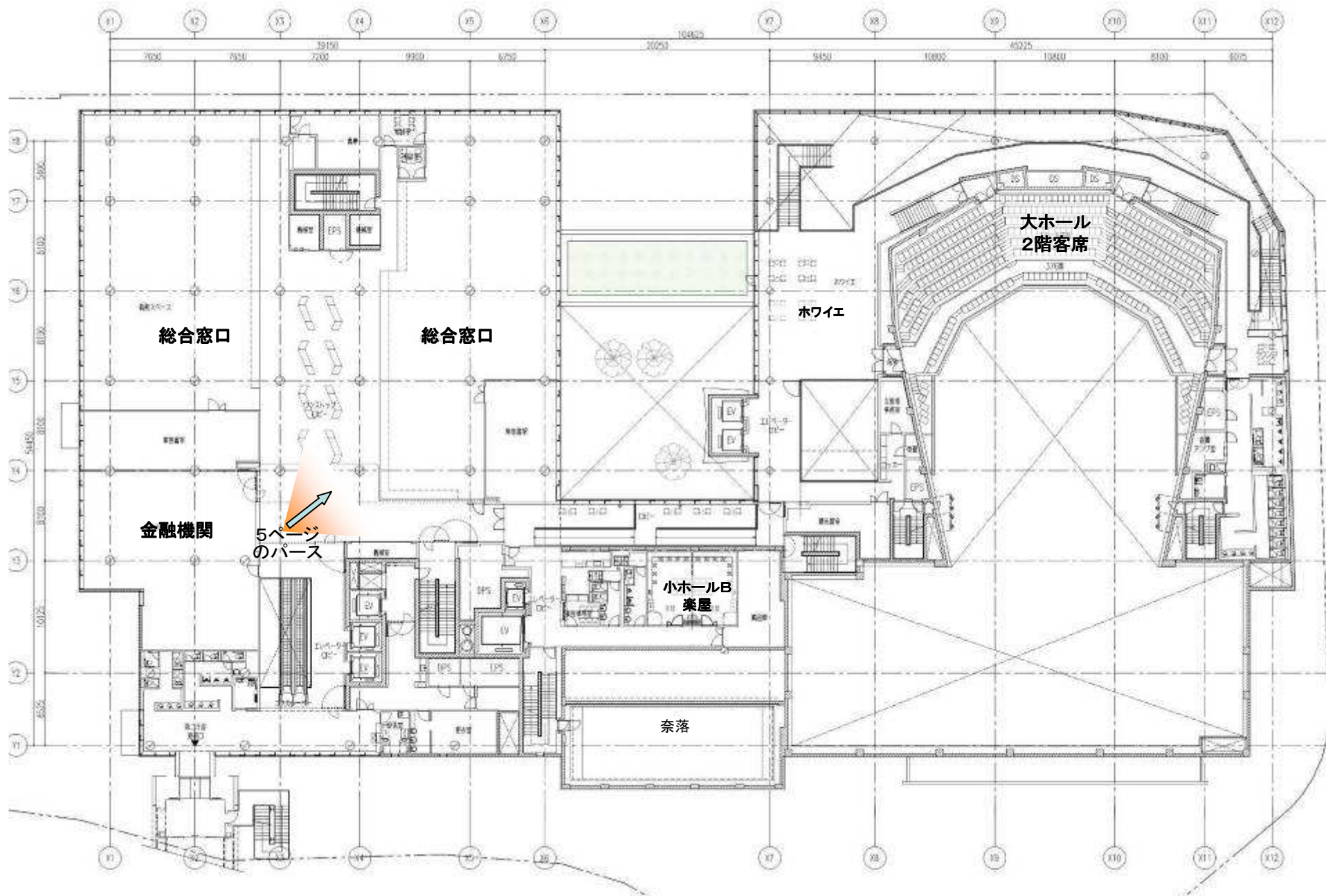
2階平面図
