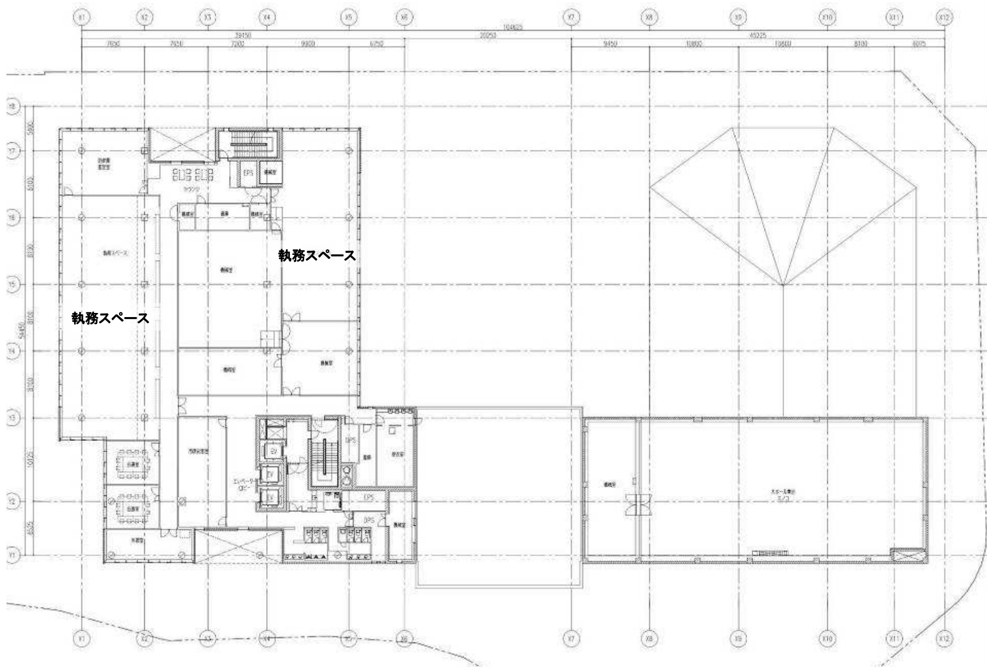
6階平面図
