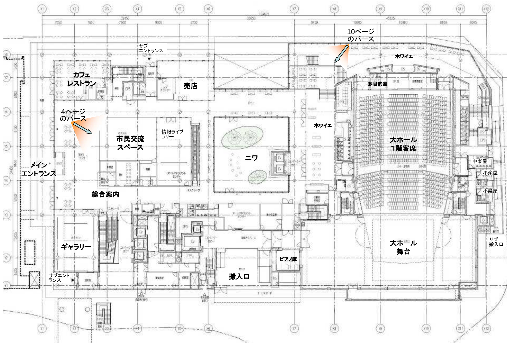
1階平面図
