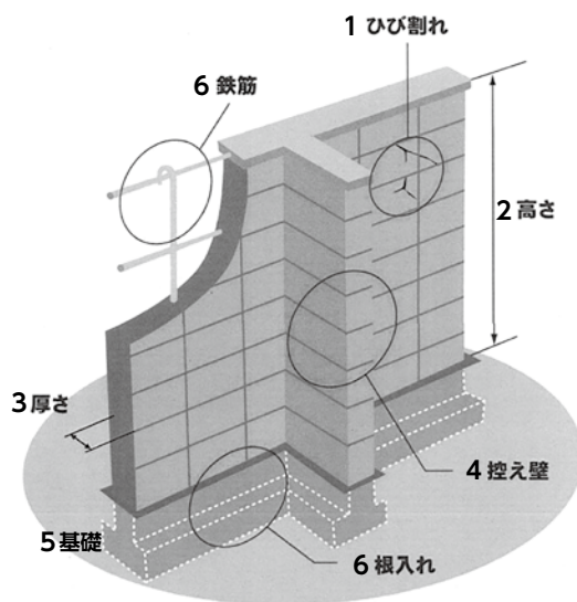
出典:パンフレット「地震からわが家を守ろう」 日本建築防災協会2013.1 より
