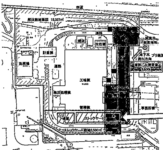
国補ストックヤード建設・旧清掃センター焼却施設解体工事の概要と場内埋設ごみ状況予想図
