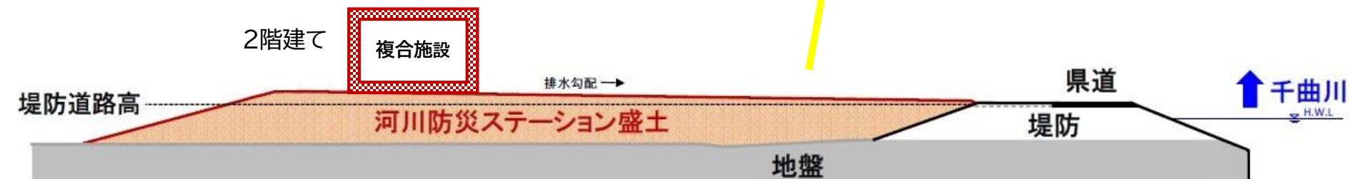
■河川の上流から下流を見る(横断イメージ)
