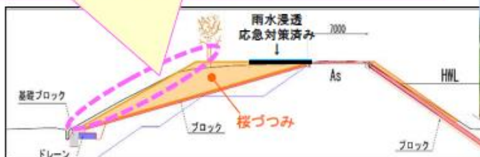
＜法面応急対策のイメージ＞
