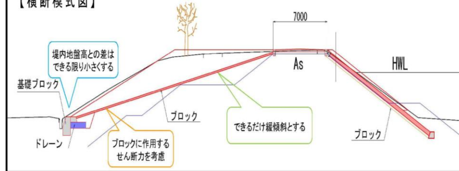
【横断模式図】
