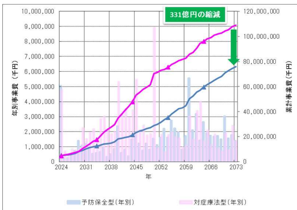
図 5-1 維持管理手法別の事業費の比較
