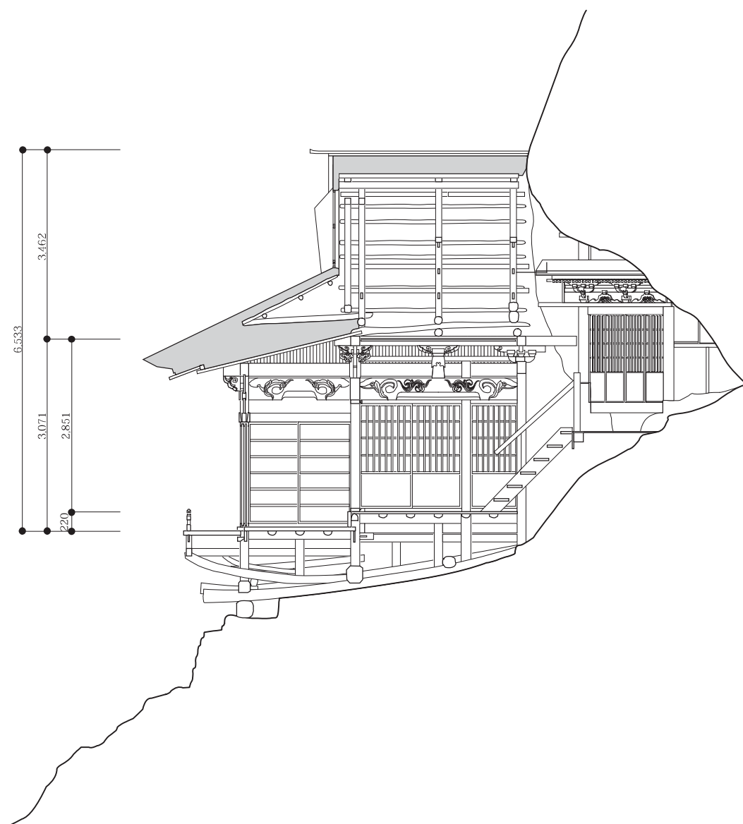
戸隠田頭の巖窟観音堂 東側断面図 (S=1/80)
